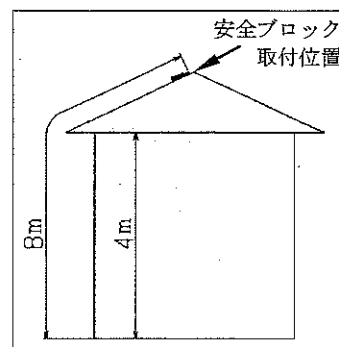
図1. 設置に必要な高さについて
