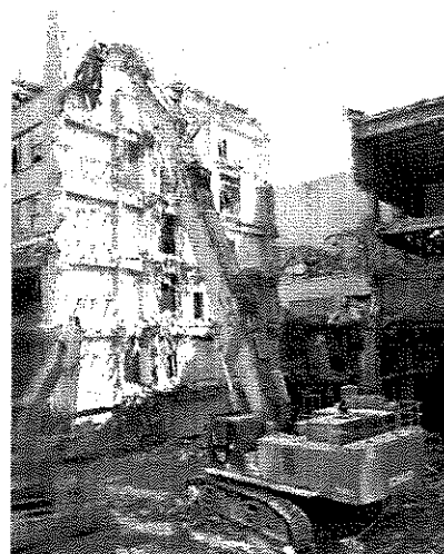
特定解体用機械のコンクリート圧碎機 コベルコ建機株式会社製、同社提供
