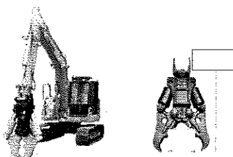
コンクリート圧砕機（コマツ製、同社提供）と アタッチメントのコンクリート圧砕具（大割）
